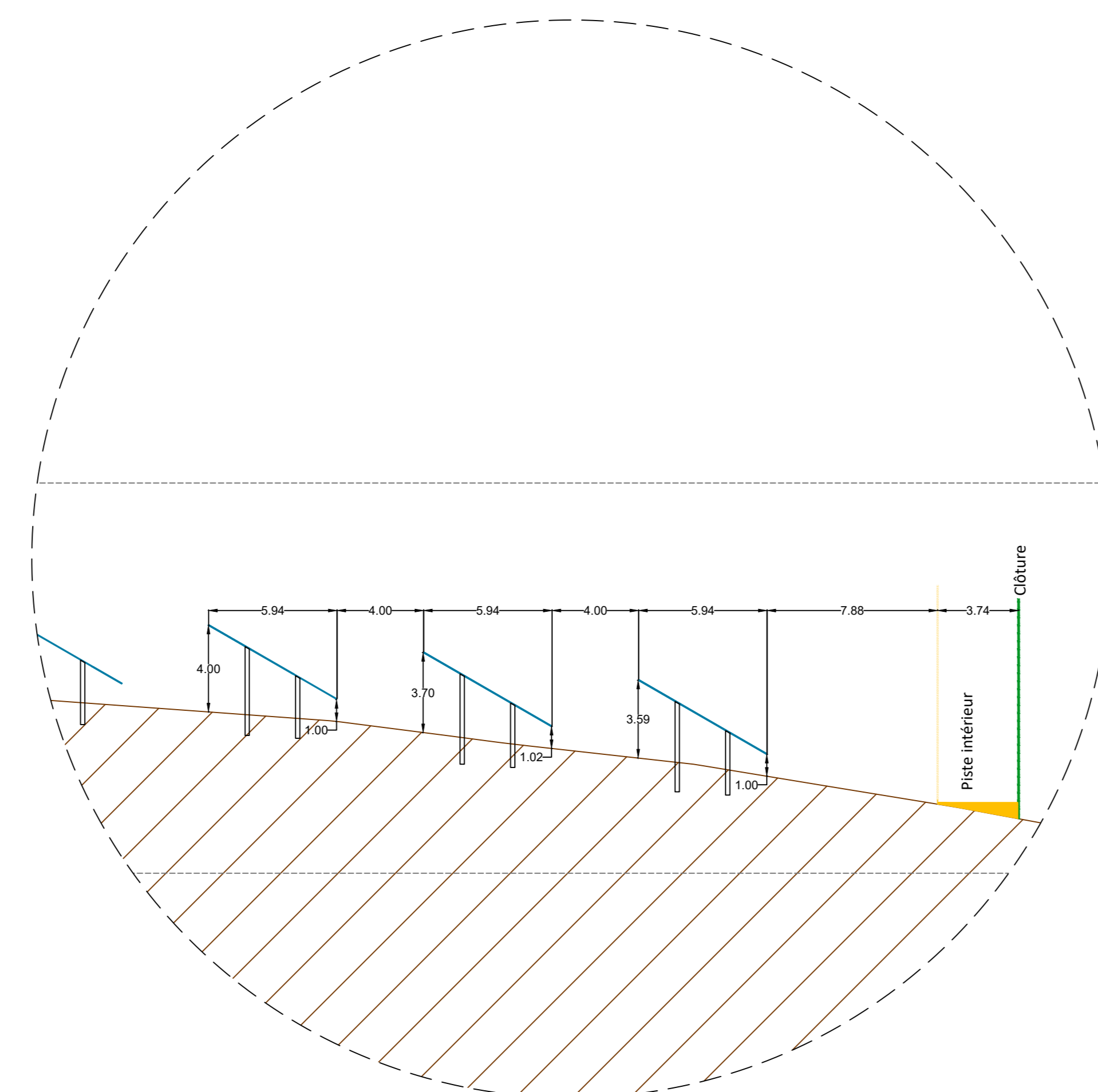
DÉTAIL 2 ÉCHELLE 5:1
