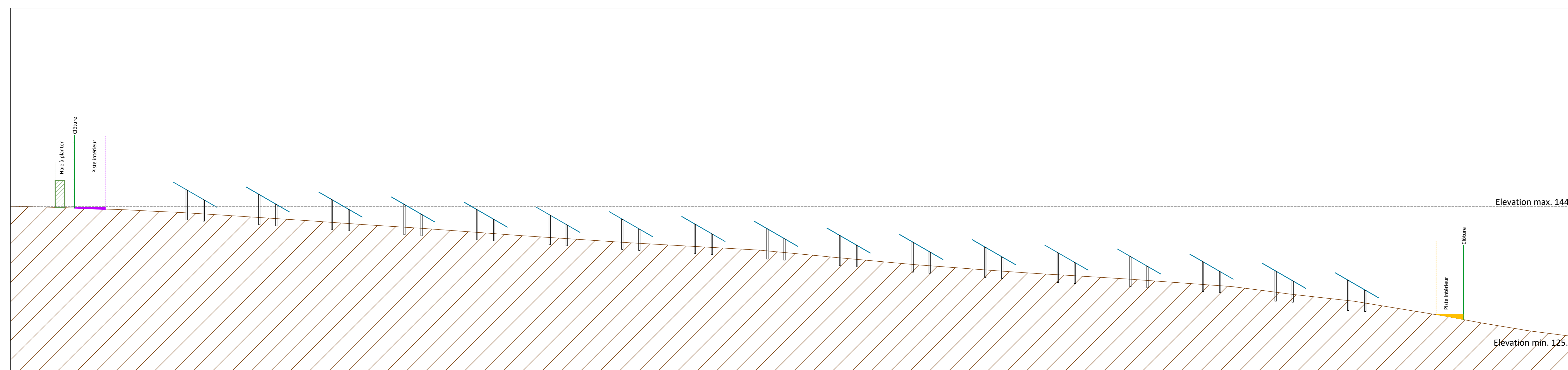
COUPE AA' ÉCHELLE 1 / 250
