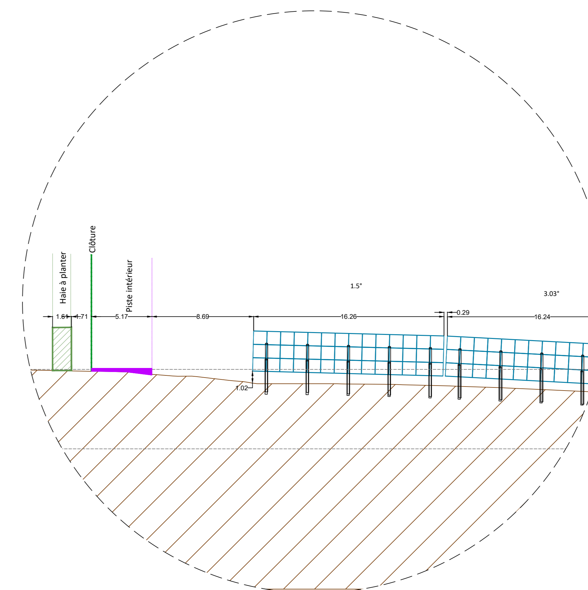
DÉTAIL 3 ÉCHELLE 5:1
