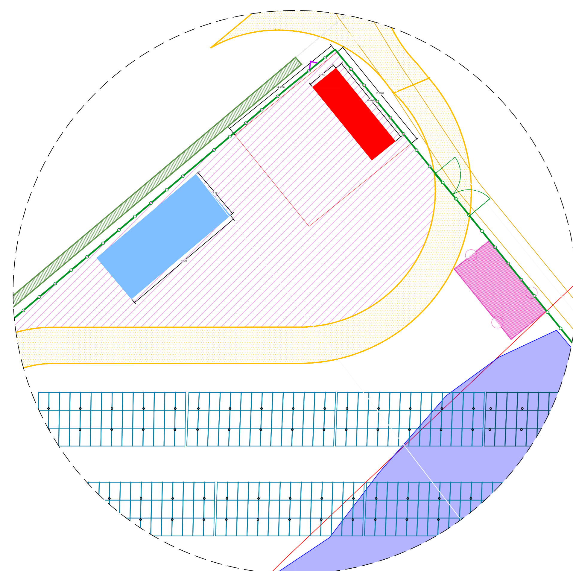
DÉTAIL 1 ÉCHELLE 1 / 250
